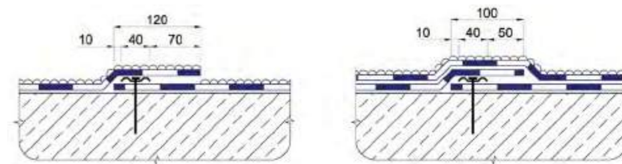
однослойная кровельная система
